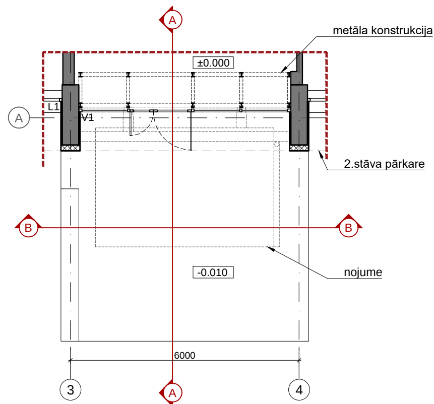
1. STĀVA PLĀNA FRAGMENTS (M1:100)
