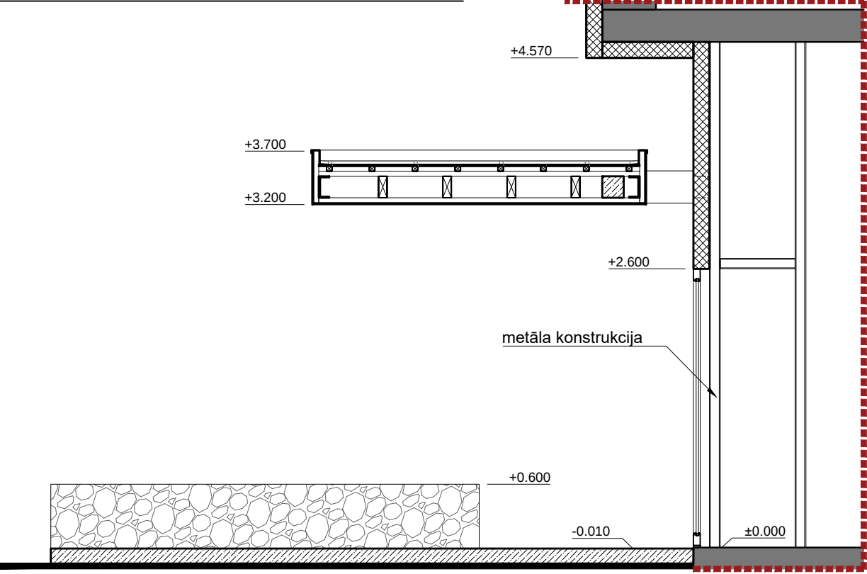
GRIEZUMS A-A (M1:50)
