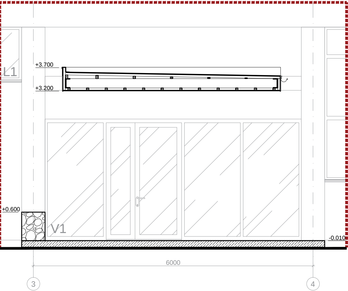
GRIEZUMS B-B (M1:50)
